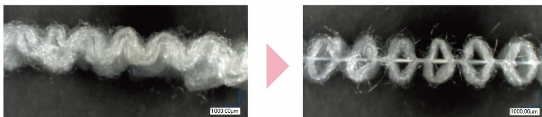
従来品断面図：ホットメルト（接着剤）接着
